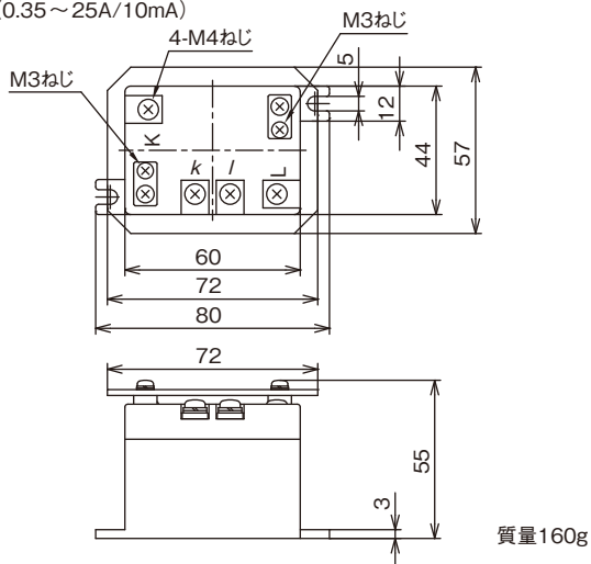
MR-CTN (0.35 ~ 25A/10mA)
