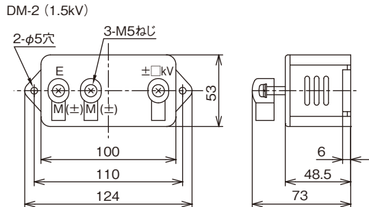
DM-2 (1.5kV)
