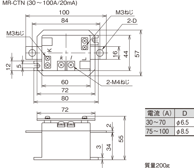
MR-CTN (30 ~ 100A/20mA)
